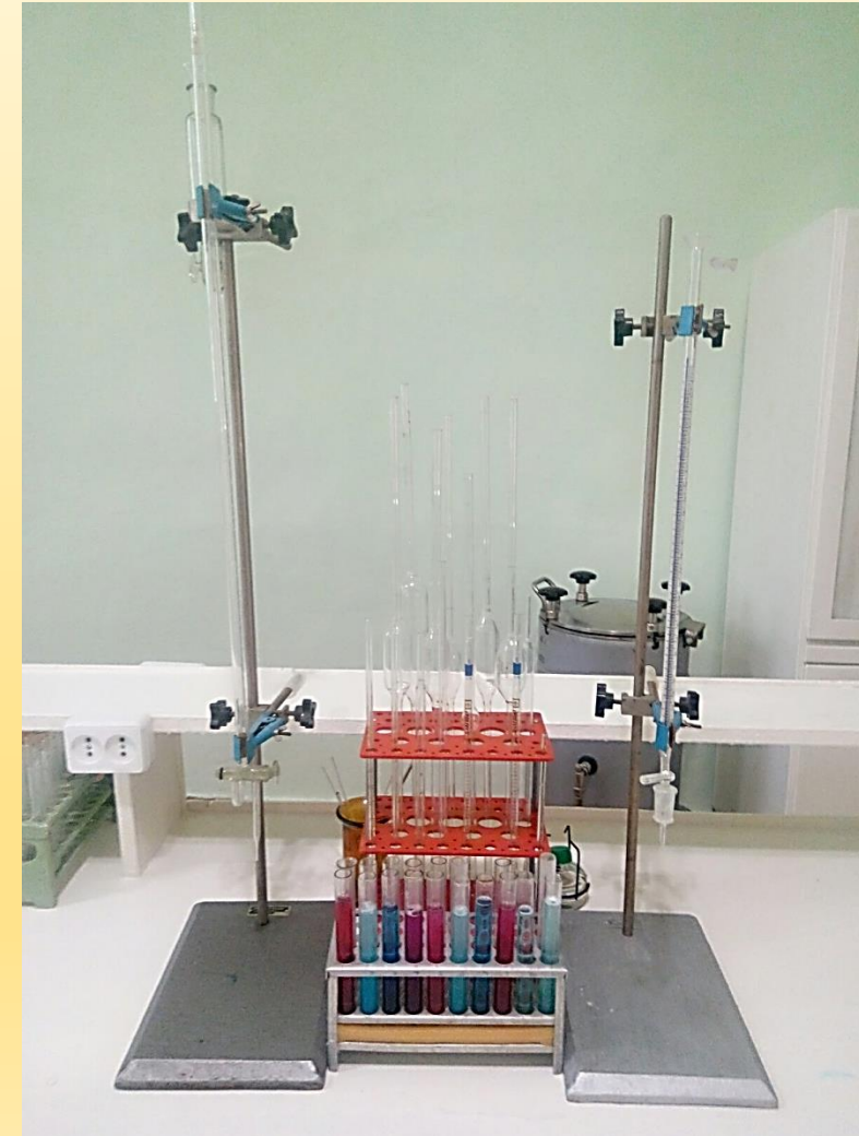
Титрувальна установка
